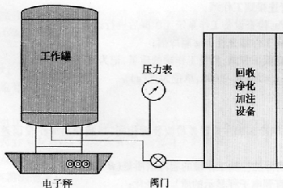
图1 制冷剂回收速度检验装置
